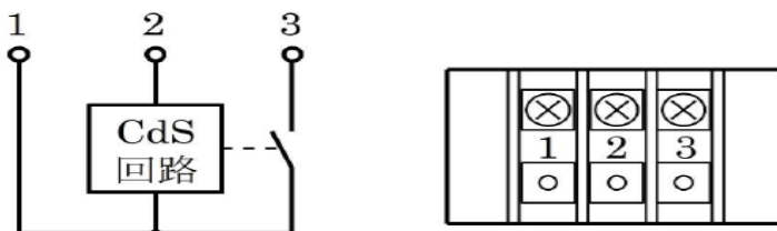
内部結線図
